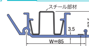
#85RW 既設管径:φ1200~1350
