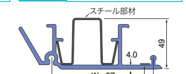
#97RW 既設管径:φ1500~1650
