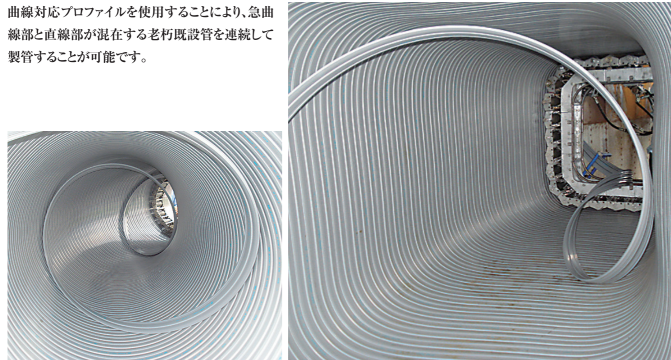
更生管径: φ840 R=4.2m (5D)
