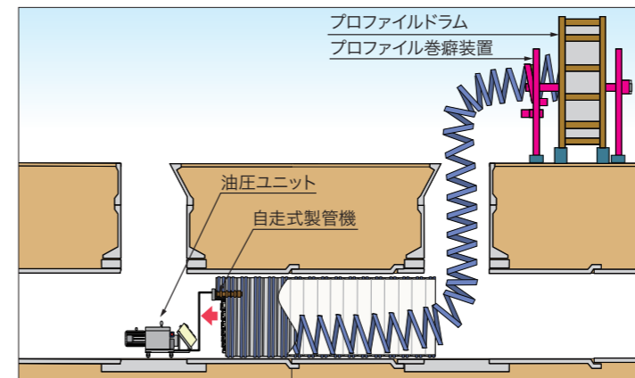
#67RW 既設管径:φ800~900
