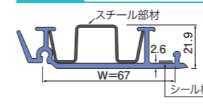
#67RW 既設管径:φ800~900
