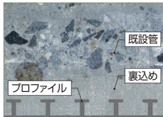
● モルタルの断面
