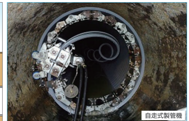
#85RW 既設管径:φ1200~1350
