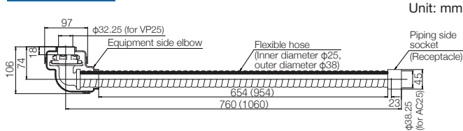
Receptacle type
