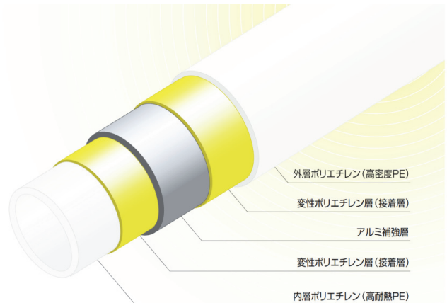
〈スーパーエスロメタックスの構造〉
