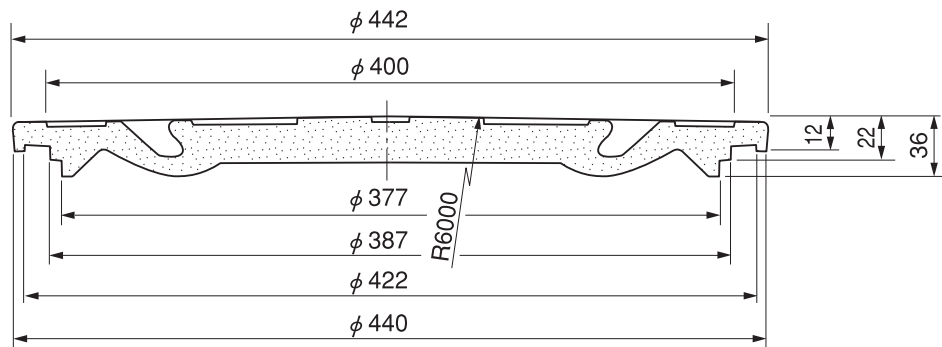
A-A'断面
