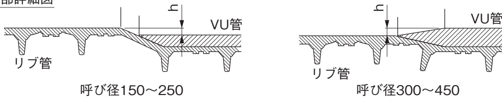
A部詳細図
