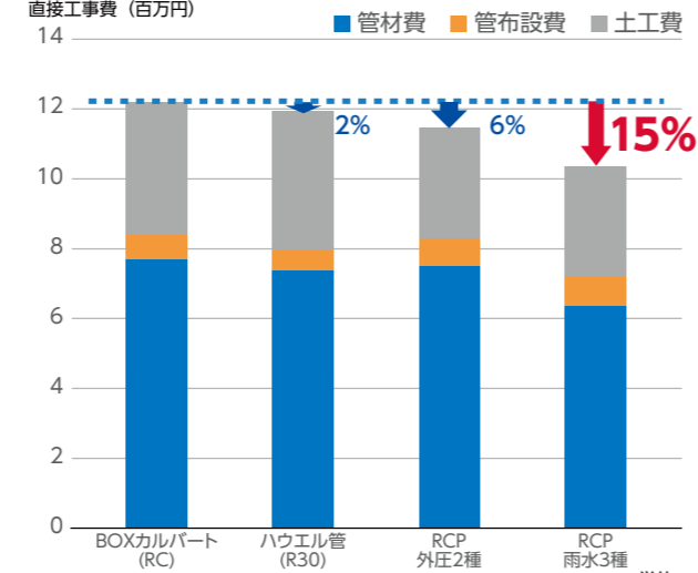
【直工費比較 呼び径1100※の場合】 ※雨水3種管 φ1350は企画中
