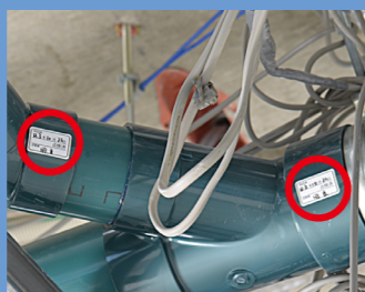
継手部に確認シールを貼付して施工管理
