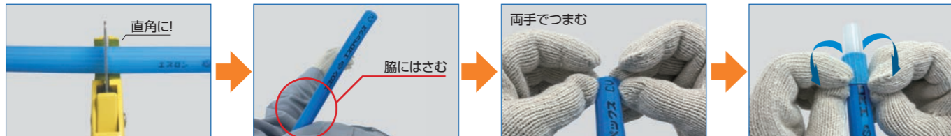
1. 被覆ごと切断 2. 脇にはさむ(近傍固定も可) 3. 両手で被覆をつまむ 4. 勢いよく一気にめくり返す(約30mm)
