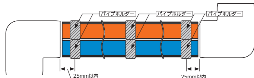
■断面図 (保温付の場合)
