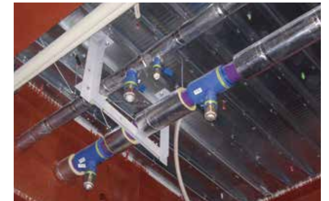
天井内配管 (ネジで分岐)
