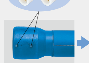
ターミナルピン 取り付け位置
