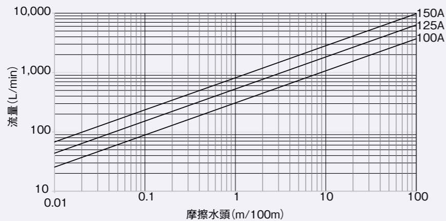
EF継手の等価管長
