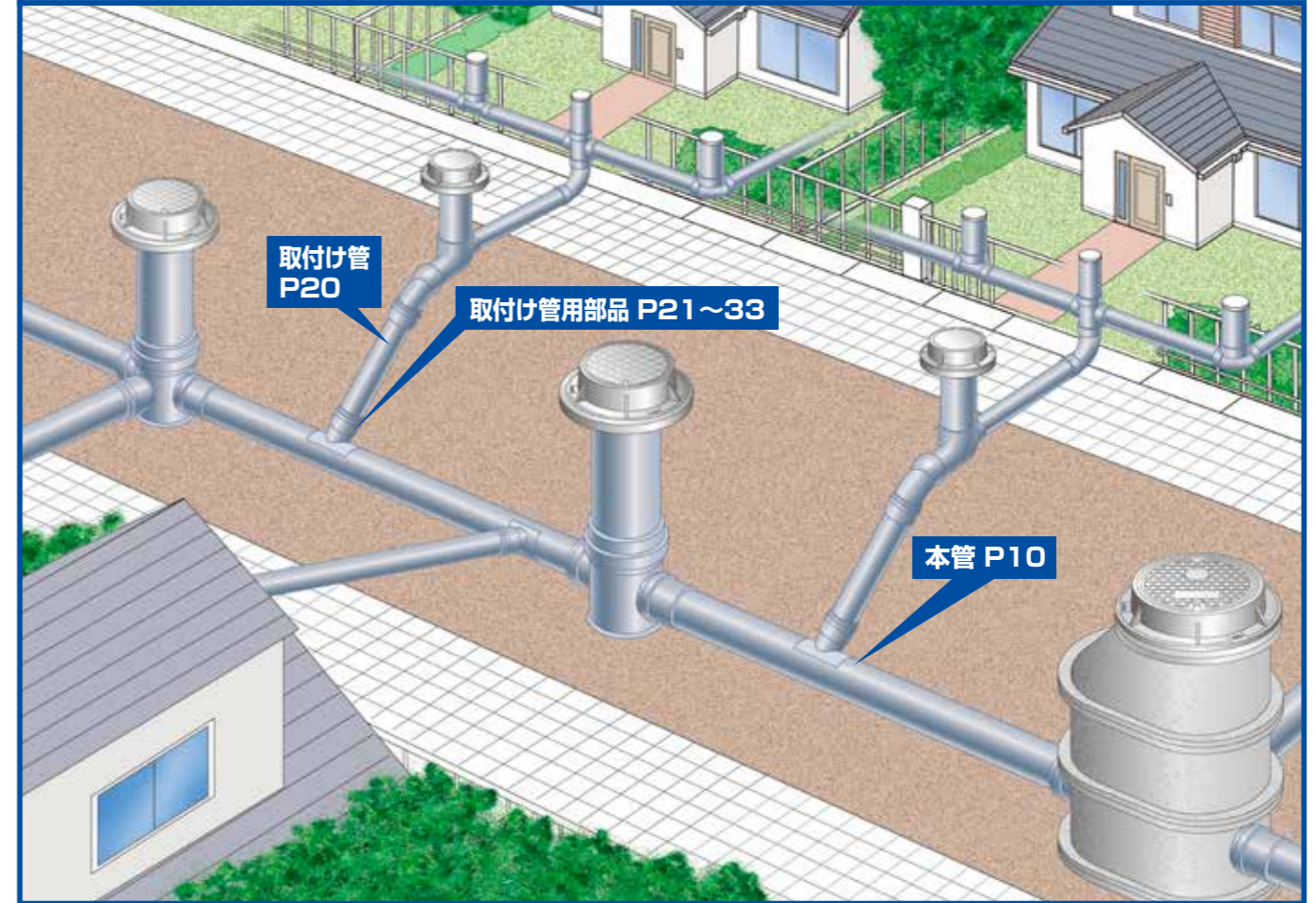
小型マンホールの場合
