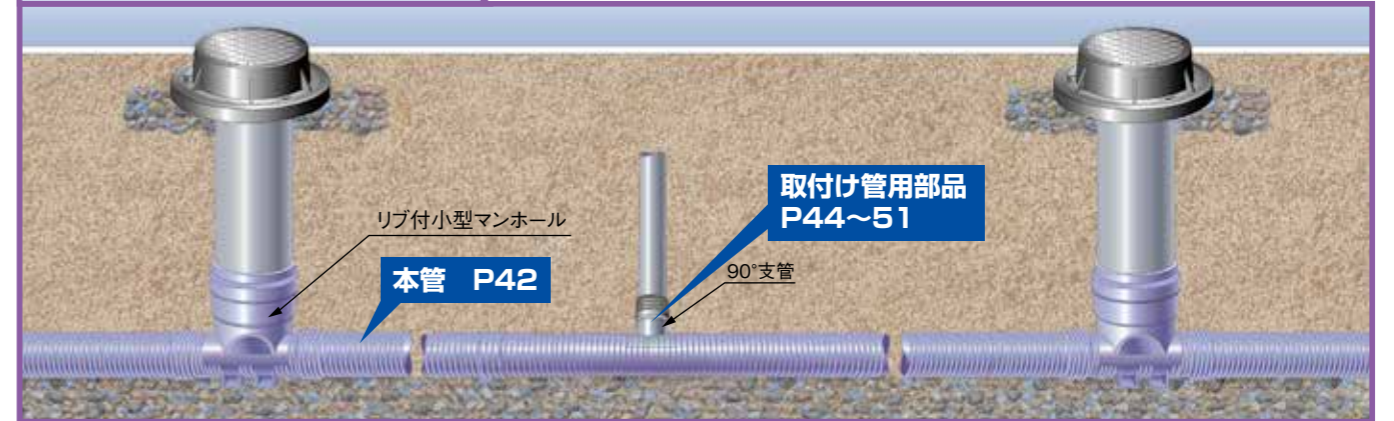
配管例
