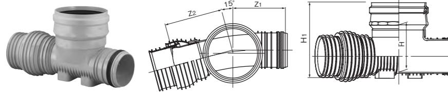
15度曲り 15L右・左-F-PRP
