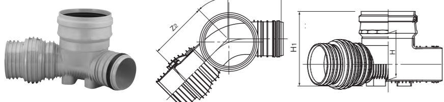
45度曲り 45L右・左-F-PRP
