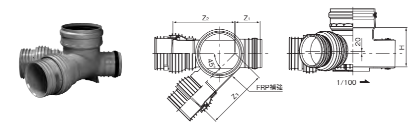
45度合流 45Y右・左-F-PRP
