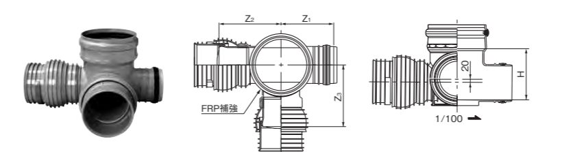
90度合流 90Y右・左-F-PRP
