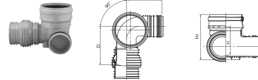
90度曲り 90L右・左-F-PRP
