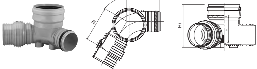
60度曲り 60L右・左-F-PRP
