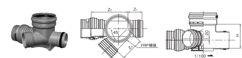
45度合流 45Y右・左-FR-PRP
