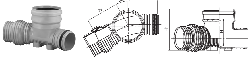
30度曲り 30L右・左-F-PRP
