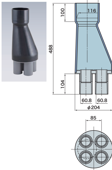
連系集約管継手本体
