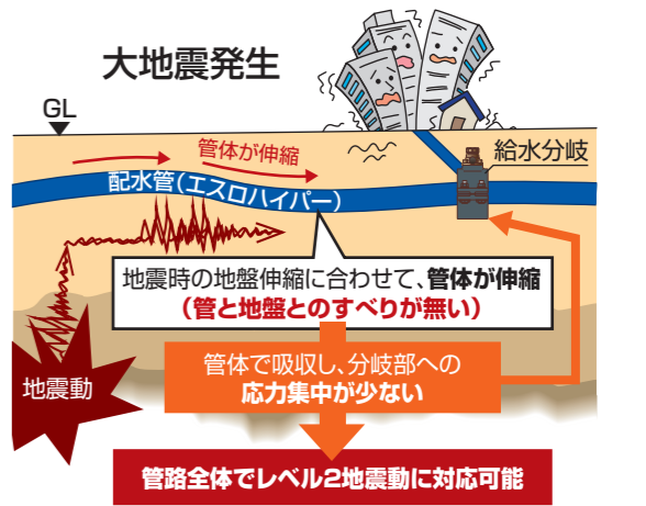
図 エスロハイパーの地震時挙動
