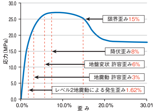
図 エスロハイパーの応力-ひずみ線図 (手引き本編 第3章: 水道配水用ポリエチレン管の性能より抜粋)
