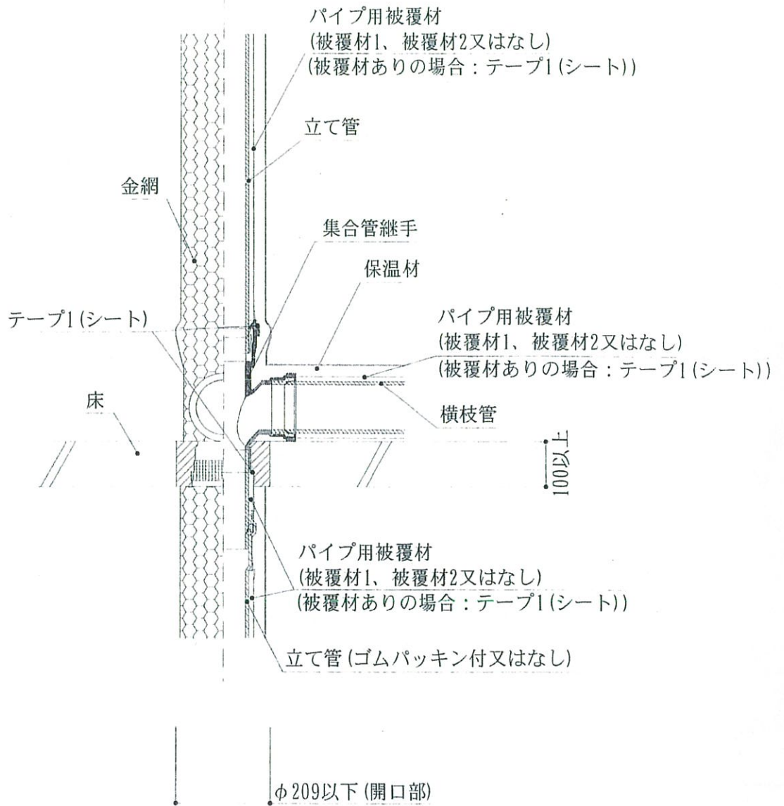
図3 配管の構造例（脚部継手を接続しない場合）
