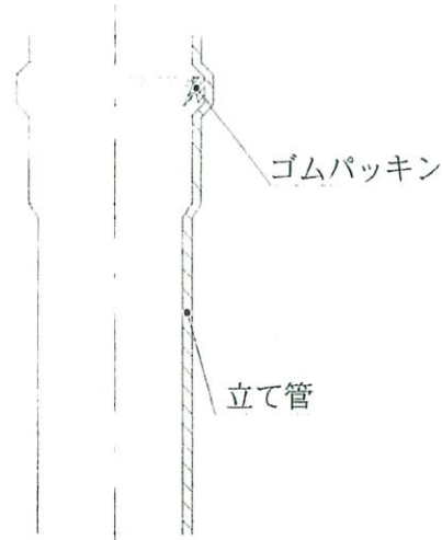
図6 立て管（ゴムパッキン付き）の構造例
