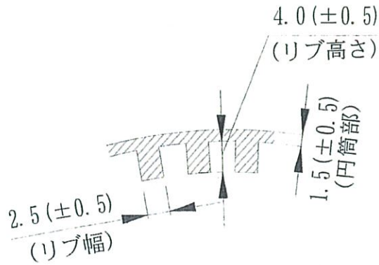
図7 パイプ用被覆材1の断面構造例
