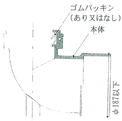
図10 脚部継手の構造例 (被覆材なし)
