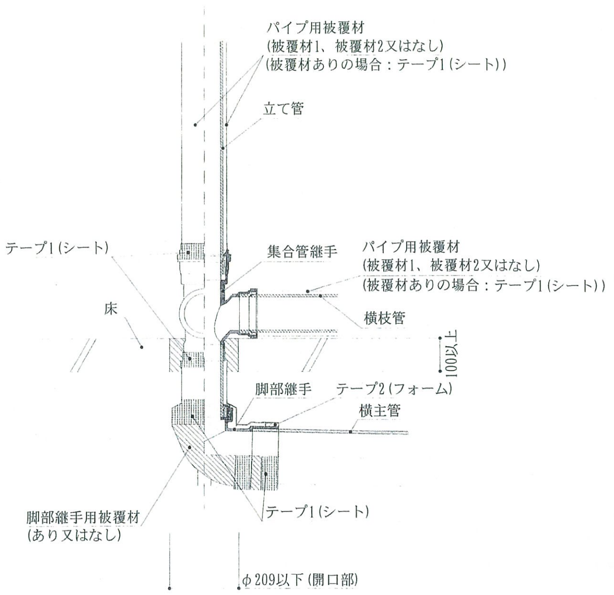
図 1 3 施工図例 (脚部継手を接続する場合)
