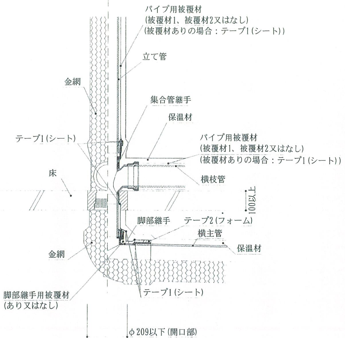
図4 配管の構造例（脚部継手を接続する場合）
