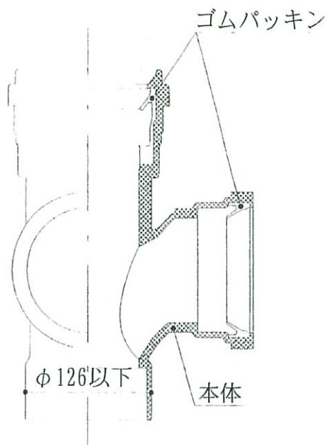
図9 排水継手の構造 (一例)
