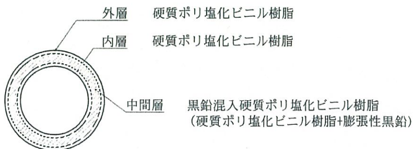
図5 樹脂製継手下部の黒鉛混入硬質ポリ塩化ビニル管の断面構造
