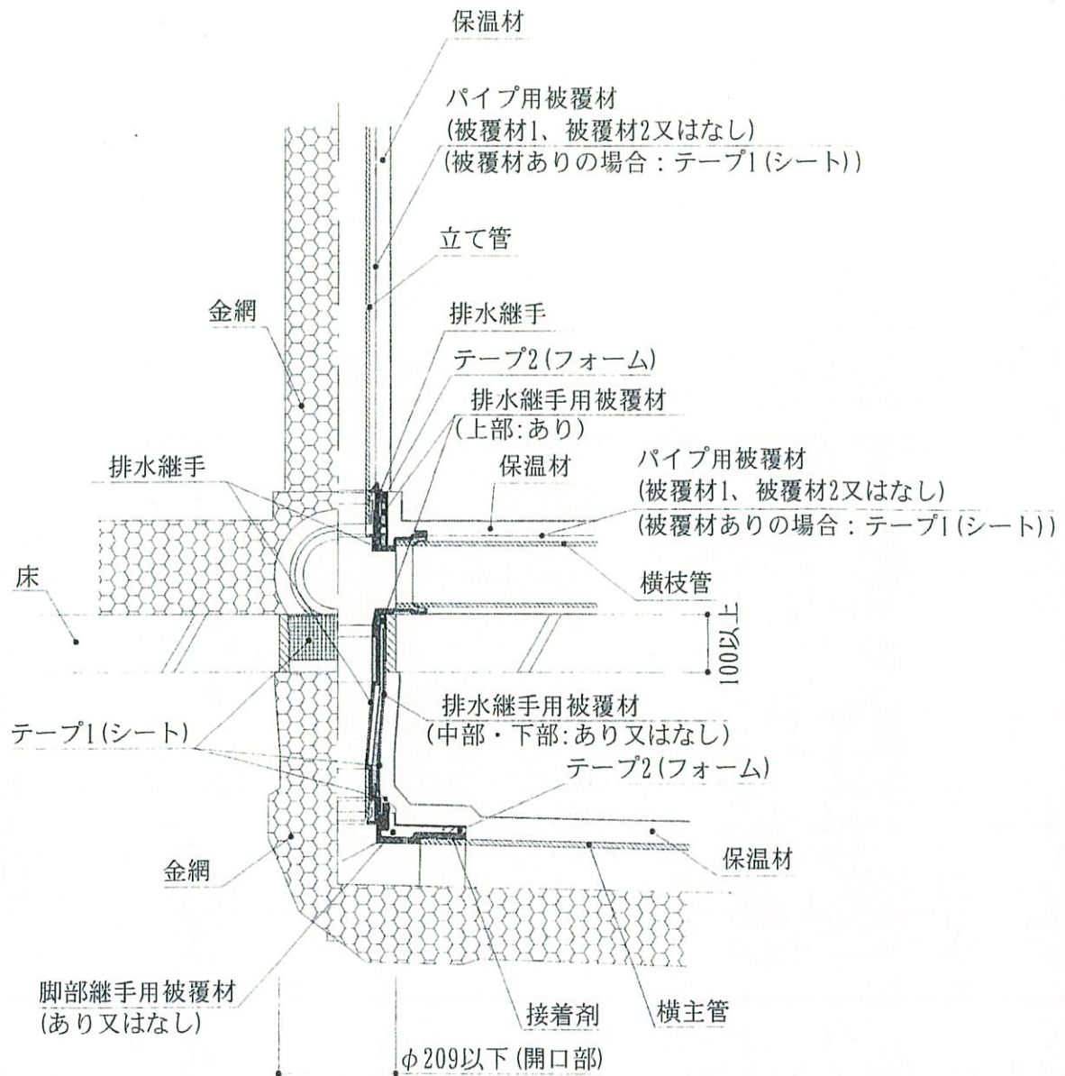
図11 施工図例(保温材を取り付ける場合)
