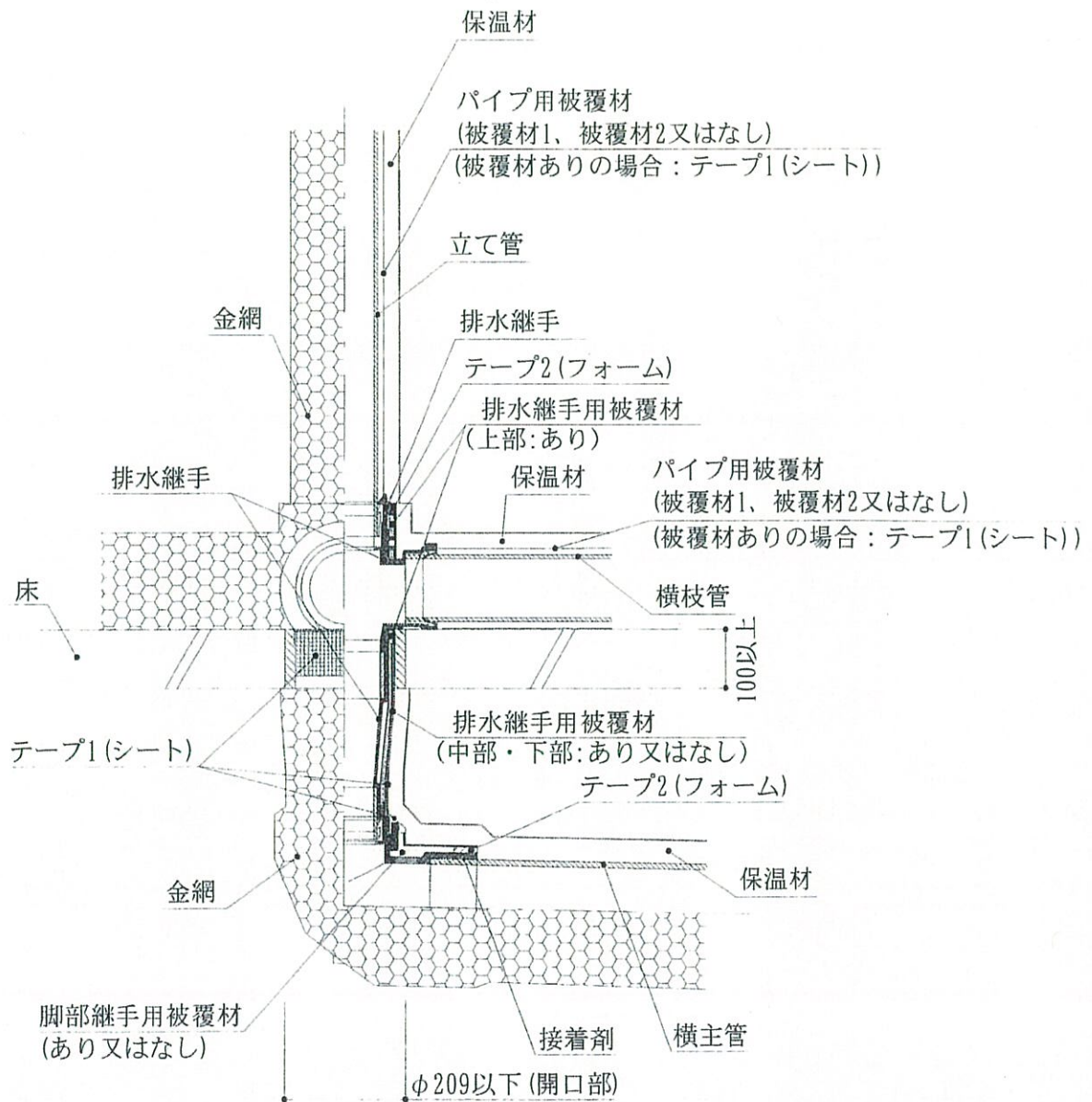
図2 配管の構造例 (保温材を取り付ける場合)
