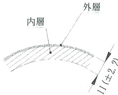
図 7 パイプ用被覆材 2 の断面構造例
