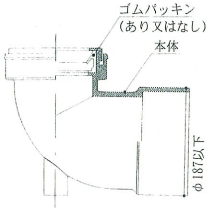
図8 脚部継手の構造例（被覆材なし）
