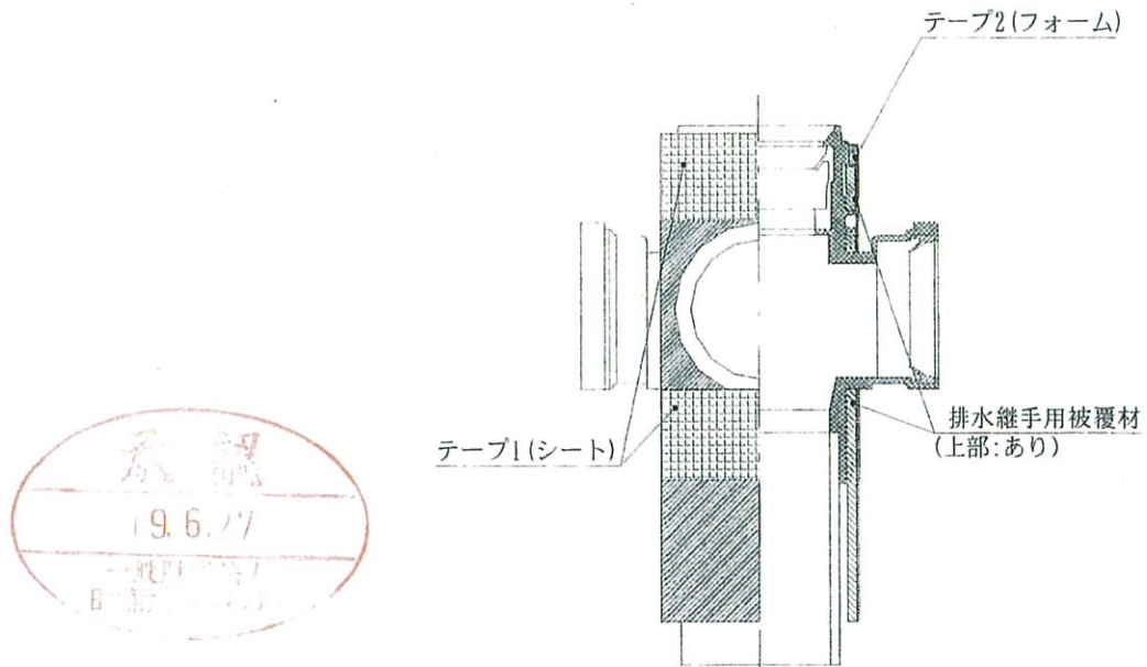
図3 排水継手の構造例
