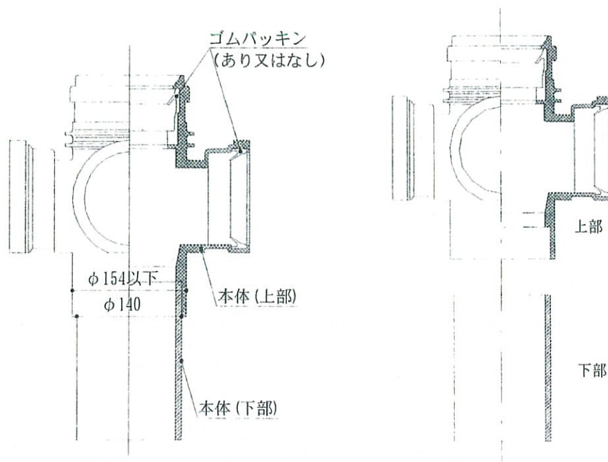
図4 樹脂製継手の構造例
