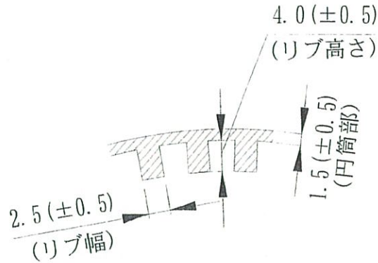
図 6 パイプ用被覆材 1 の断面構造例
