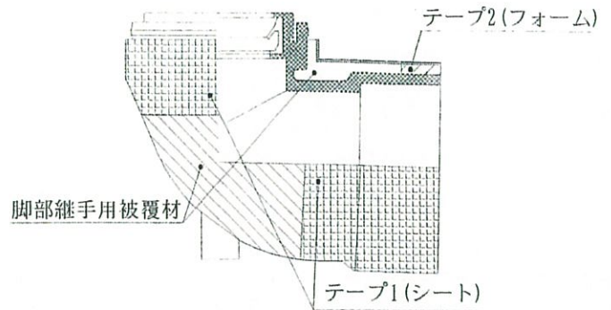
図9 脚部継手の構造例（被覆材あり）
