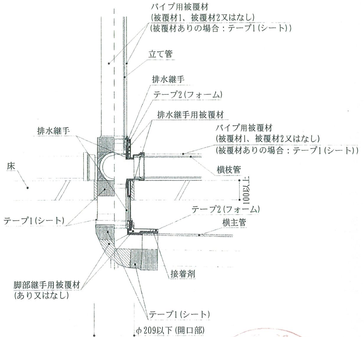
図1 配管の構造例
