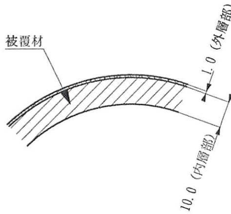
図3 被覆材の断面構造
