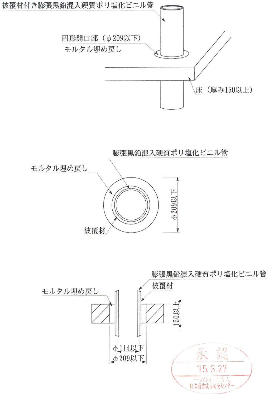
図4 施工図例
